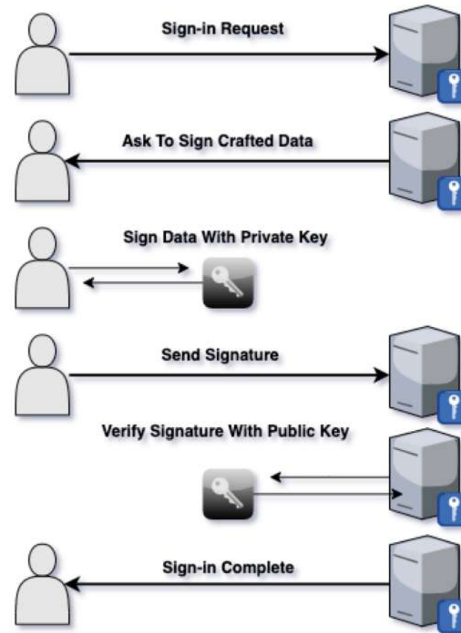
Login Flow
